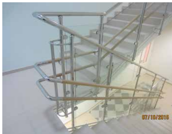
Ограждение в школе с торцевым креплением и большим выносом стоек относительно лестничного марша в целях сохранения ширины лестницы по пожарным нормам. Расстояние между стойками и торцом марша закрыто двумя ригелями.
