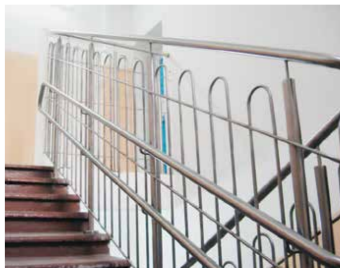
Самый бюджетный вариант детских ограждений с установкой стоек сверху в ступень. Горизонтальные направляющие из трубы Ф16мм, вертикальное заполнение - согнутая труба Ф16мм, приваренная внахлест с внутренней стороны марша.
