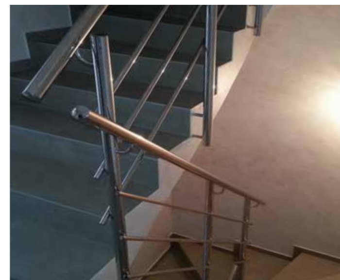
Боковой крепеж трехригельного ограждения в условиях малого пролета между маршами (70 мм). Вынос на прутках возвращает поручень в плоскость марша. Стойки вынесены на 50 мм относительно торца плоскости марша.
