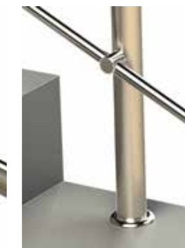
Крепление ригеля через ригеледержатель k018.
