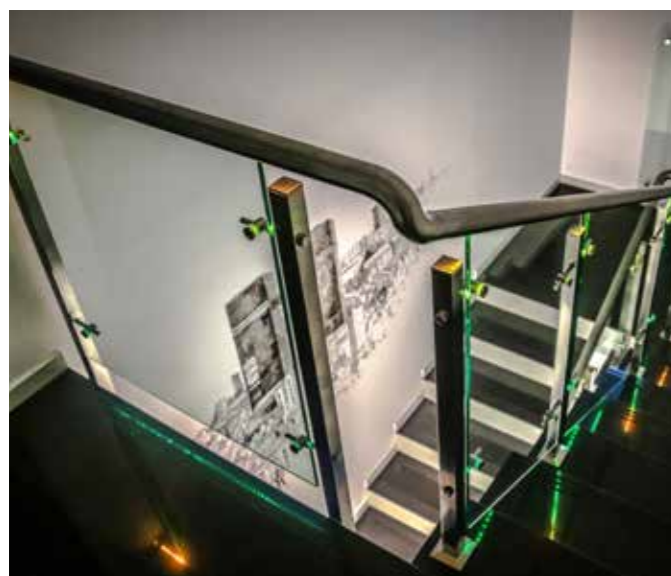
Уникальное решение освещения стекла непрерывной линией с помощью подсветки, встроенной в поручень, меняющей цвет.
