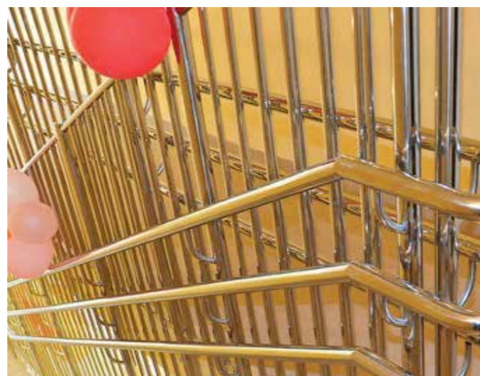
Ограждения в ясли для самых маленьких с тремя поручнями на высоте 500мм, 700мм и 900мм. Вертикальное заполнение из трубы Ф25мм. Относительно высокая стоимость ограждения из-за большой металлоемкости и трудоемкости.
