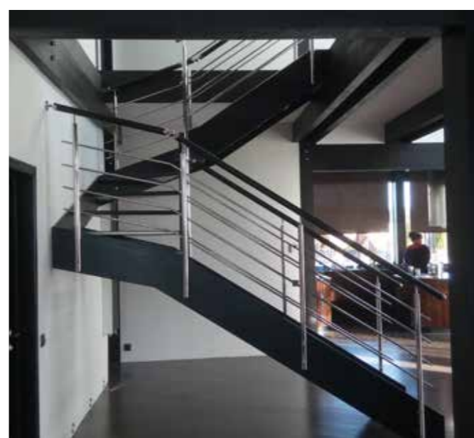
Торцевое крепление стоек ограждения к несущей тетиве лестницы, поручень ПВХ черного цвета закреплен в стену через фланец k245. Заполнение из 4-х ригелей продиктовано динамичным дизайном.
