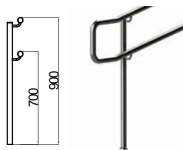
Вариант исполнения ограждений №1: поручни на высоте 900 мм и 700 мм на выносе относительно стойки.
