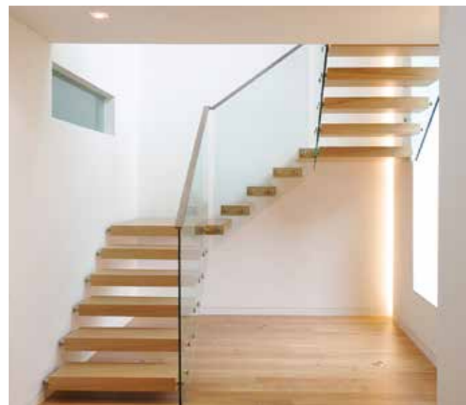
Красивая консольная лестница с ограждением без стоек и торцевым креплением. Подсветка эркера лестницы с помощью светильников, встроенных в угол лестницы.
