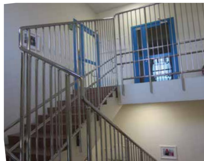
Ограждение с ригелями в детском саду для детей с отставанием в развитии. Выполнено с тремя поручнями д.38 мм на высоте 500 мм, 700 мм и 1500 мм по ГОСТу. Поручни завязаны между маршами. Из за бокового крепежа и колодезного типа лестницы, при повороте на 90 градусов образуется выход на вертикаль высотой в 1 высоту ступени.
