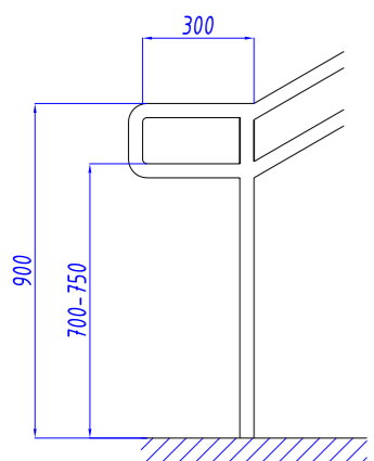
Окончание пандуса для инвалидов по ГОСТ Р 51261-99.
