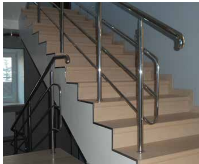
Поручень уменьшенного диаметра (38 мм) для удобного хвата, ригели завязаны травмобезопасно. Наконечник k006, минимальная крышка основания стойки k035. Отвод оконечный с полукруглой заглушкой.
