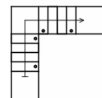
Ригельное ограждение с выходом в горизонт, поручень и ригели развязаны.
