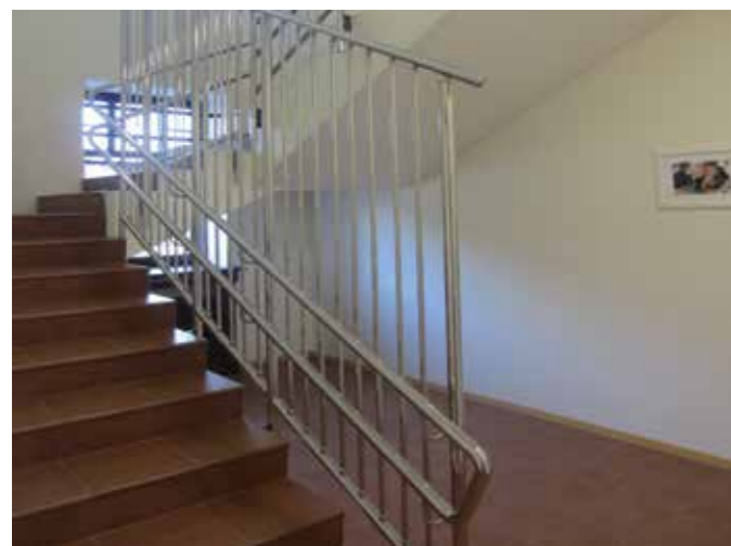
Ограждение с ригелями в психоневрологическом детском центре. Выполнено с тремя поручнями д.38 мм на высоте 500, 700 и 1800 мм по ГОСТу. Поручни завязаны между маршами, на конце каждого поручня закольцовка. Из-за колодезной лестницы при повороте на 90 градусов образуется выход на вертикаль.
