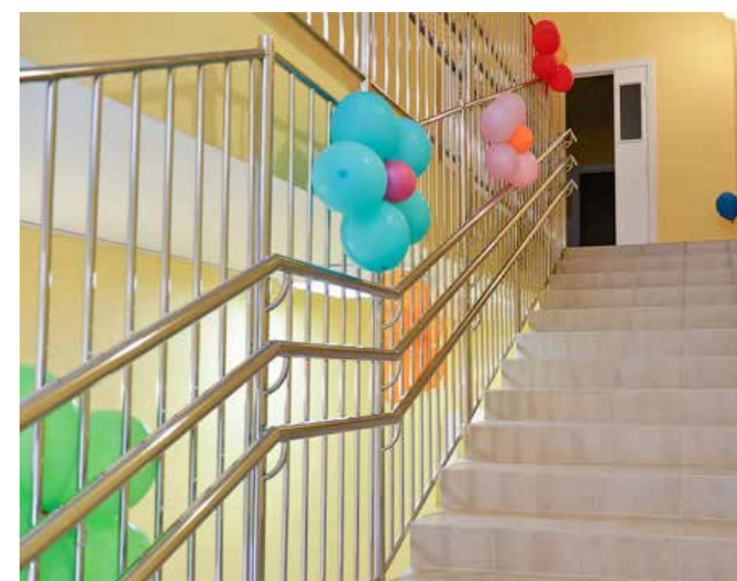
Ограждение с вертикальным заполнением в школе для всех классов. Выполнено с тремя поручнями д.38 мм на высоте 500 мм, 700 мм и 1500 мм по ГОСТу. Поручни повторяют геометрию лестничного марша. Стойки закреплены в торец лестницы, чтобы сохранить ее ширину по пожарным нормам.
