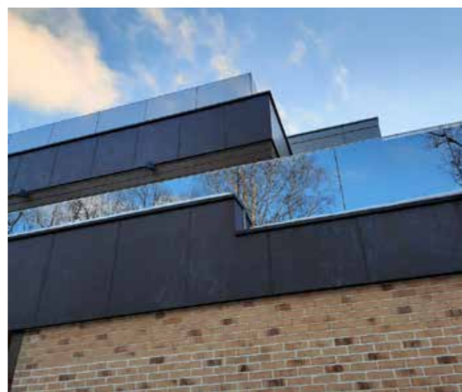
Ограждение многоуровневых балконов стеклом 8+8мм стопсол триплекс цвета бронза/серое в массе и креплением в зажимной алюминиевый профиль.
