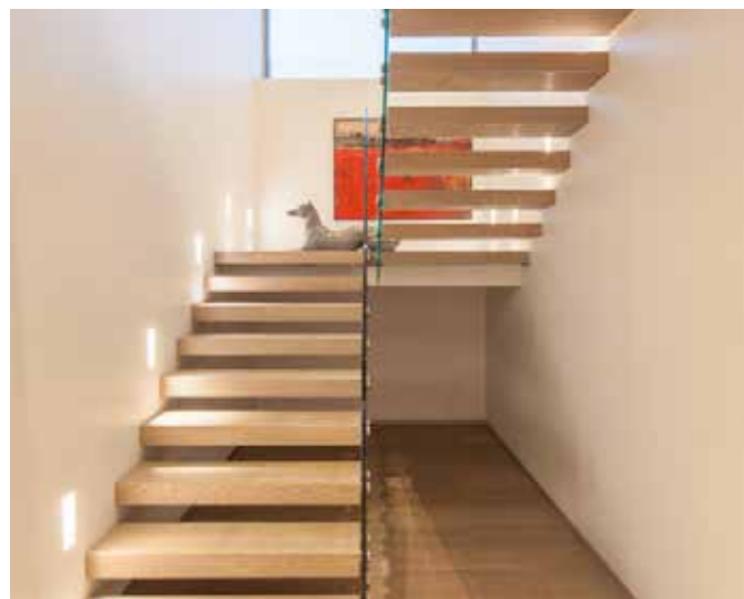
Консольная лестница со ступенями 70мм из дуба с цельностеклянными ограждениями без поручня, закрепленными в торец ступеней.
