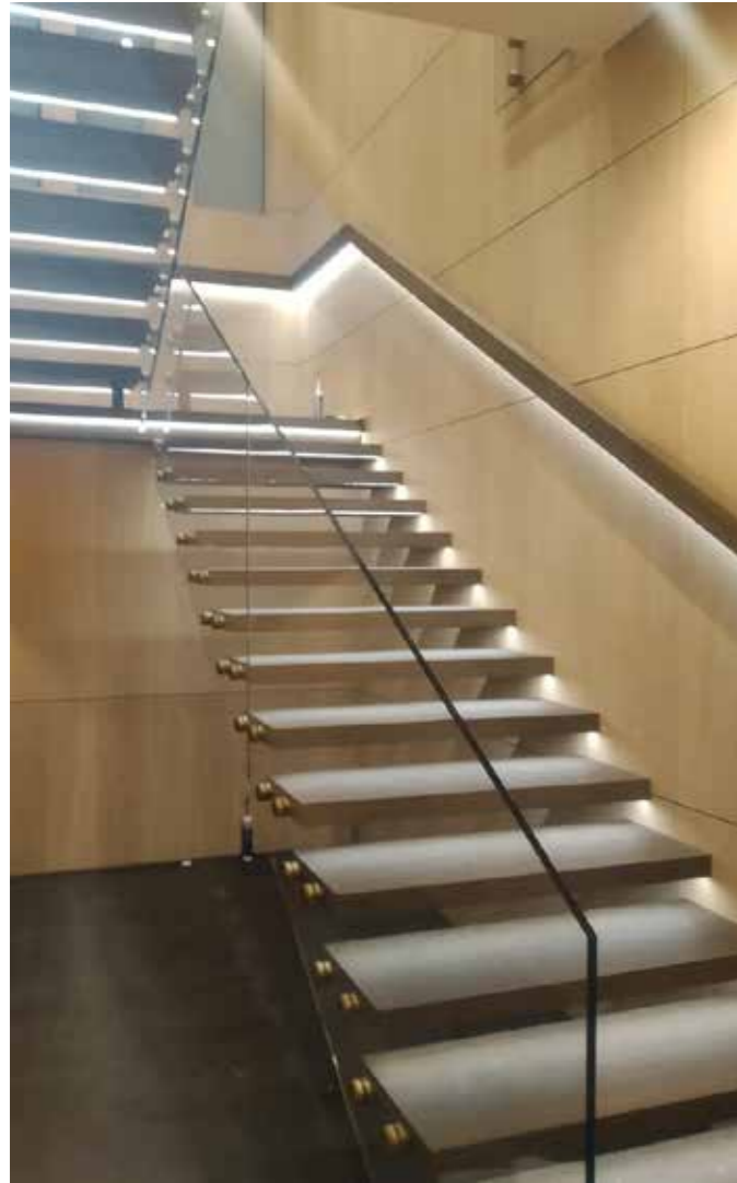
Стекланные перила толщиной 8+8мм без поручня, точечные крепления под золото.
