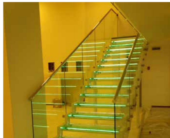
Лестница на двух косоурах из черного металла. Ступени из триплекса 10+10+10 мм с подсветкой. Ограждение из стекла 12 мм установлено сбоку. Поручень д. 48 мм с пазом.
