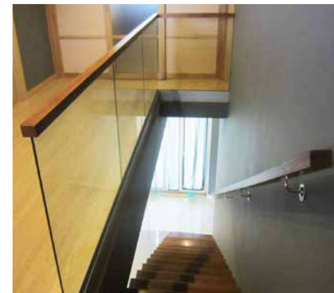
Дубовый поручень 40x60мм установлен сверху на стекло на площадке 2-го этажа и на выносных пристенных держателях по всей длине лестничного марша.
