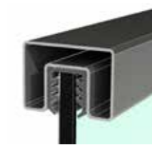
Поручень из профильной нержавеющей трубы с пазом под стекло или LED подсветку
