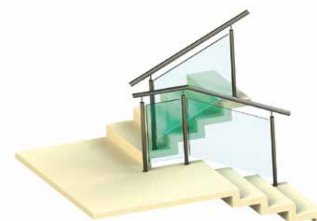
Поручень не завязан, просвет между стойками не закрыт. Применимо для маршей с просветом менее 120 мм.
