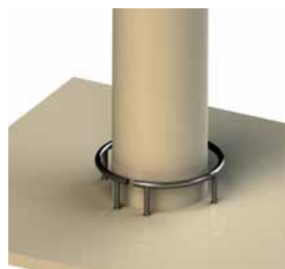
Колесоотбойник вокруг колонны (защищает облицовку от тележек).
