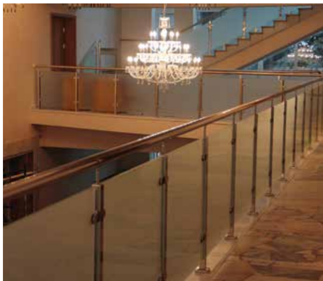
Ограждения балкона на квадратных стойках 40x40 мм. Наконечник стойки k239, крышка k076. Стекло матовое 8 мм, шаг стоек 1 метр, поручень 50 мм.
