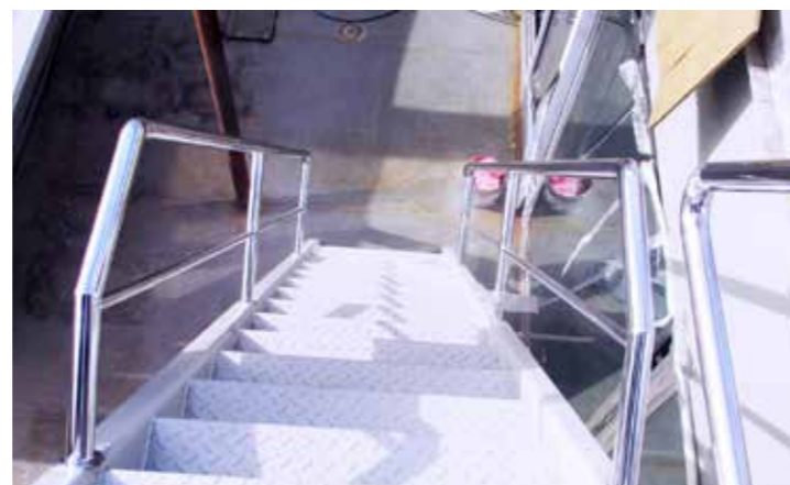
Катамаран серии ТМ-20 плавучий дом. Среди выполненных работ: леера кормовой части первой палубы с калитками и леера надстройки, кранбалки с лебедками на корме, декоративные трубы дымохода (надстройки), трап и леера с левой палубы на надстройку из нержавеющей стали.
