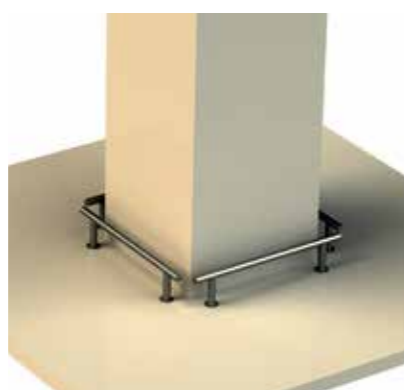
Колесоотбойники вокруг квадратной колонны, все развязано.
