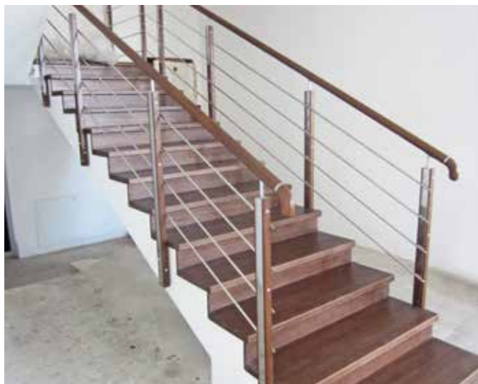
Стойки из шлифованной нержавеющей стали с боковым крепежом, со вставками из дерева, с деревянным поручнем 40 мм и оконечным деревянным отводом в цвет ступеней.
