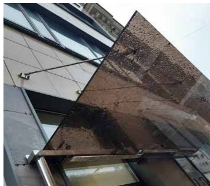
Козырек с обратным уклоном и отливом из нержавеющей стали с креплением к вентфасаду здания.
