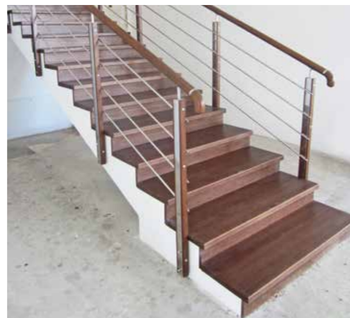
Ограждения в частном доме с ригелями, эксклюзивными стойками и деревянным поручнем с торцевым креплением по обе стороны марша для сохранения полезной ширины лестницы.
