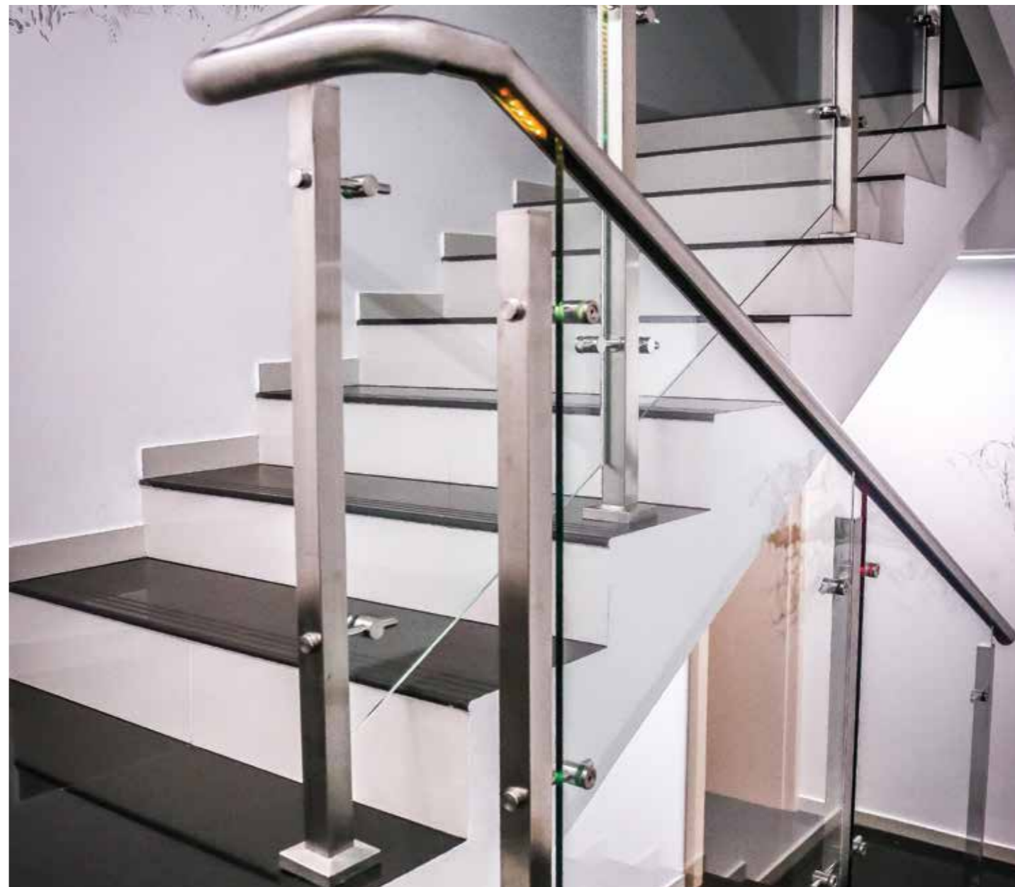
Ограждение на стойках 40x40 мм на спайдерных стеклодержателях и встроенной LED подсветкой (подробнее см. страницу 70).
