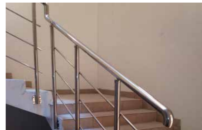
Боковой крепеж трехригельного ограждения на k056. Стандартный подскок на высоту одной ступени и сложная завязка в трех плоскостях круглого поручня диаметра 50 мм.
