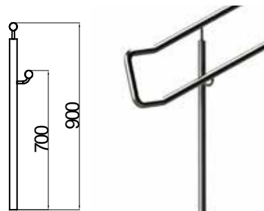
Вариант исполнения ограждений №2: поручни на высоте 900 мм сверху на стойке, поручень 700 мм на выносе относительно стойки.
